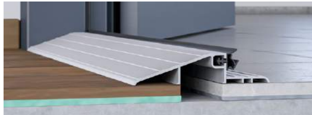
Aluminiumschwelle
