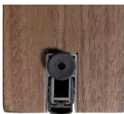
automatic bottom door seal
