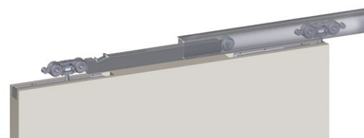
hydraulický zpomalovač
