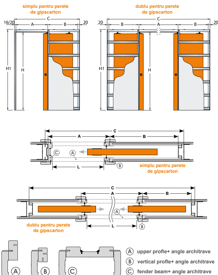
DIAGRAMA LOCALIZĂRII ELEMENTELOR DE CADRU PENTRU SISTEMUL DE GLISARE (perete de gipscarton)
