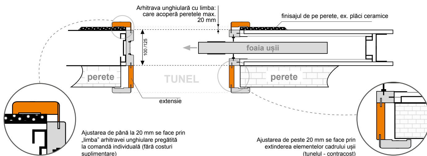
DIAGRAMA LOCALIZĂRII ELEMENTELOR DE LĂRGIRE A CADRULUI UȘII PENTRU SISTEMUL DE GLISARE „BUZUNAR”
